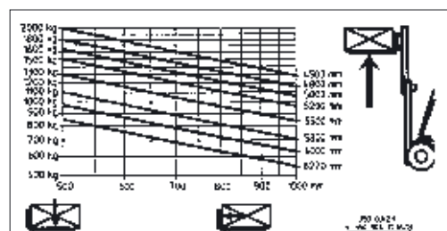
Figura 2: ogni carrello elevatore deve recare ben visibile il diagramma della portata.
