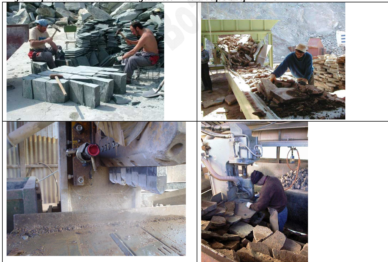
Fig.3-4: spaccatura a macchina con getti nebulizzati d'acqua e aspirazione
