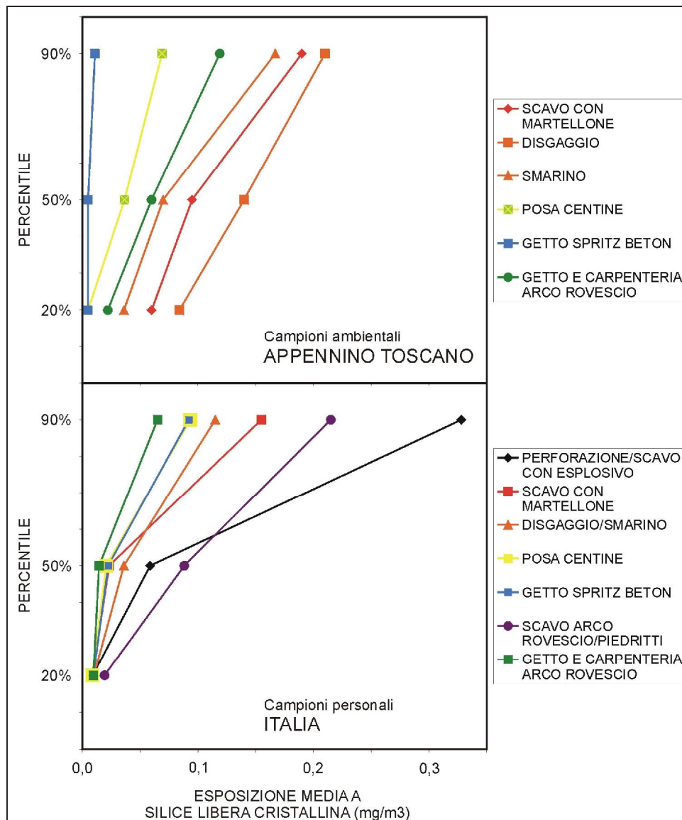
ESPOSIZIONE MEDIA A SILICE CRISTALLINA RESPIRABILE PER FASE DI LAVORO: 20°, 50° E 90° PERCENTILE. DATI RELATIVI AI CANTIERI ITALIANI E AI CANTIERI TAV DELL'APPENNINO TOSCANO
