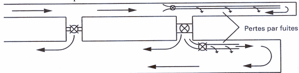
Fig. 3 Ventilation par circulation d'air avec galerie latérale: ventilation par les galeries de liaison. La galerie latérale alimente le tunnel en air frais
