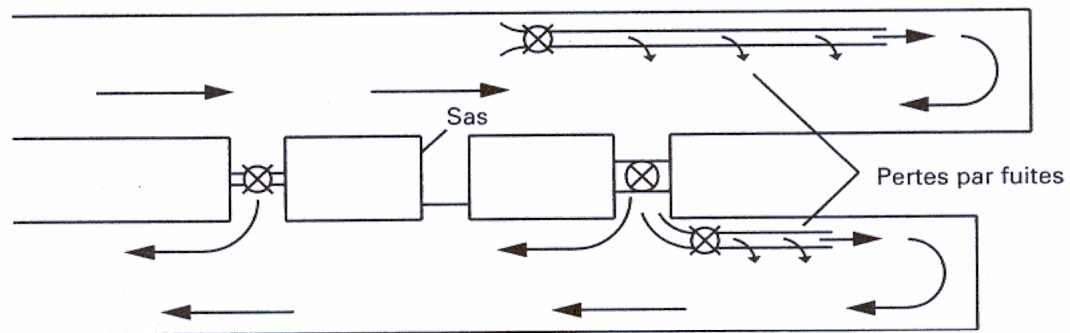
Fig. 4 Ventilation par circulation d'air de deux tunnels parallèles avec ventilation par les galeries de liaison
