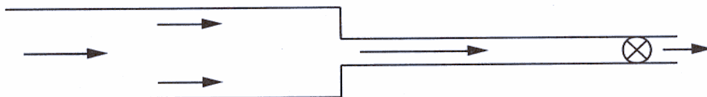
Fig. 5 Ventilation par circulation d'air dans une galerie pilote percée au préalable
