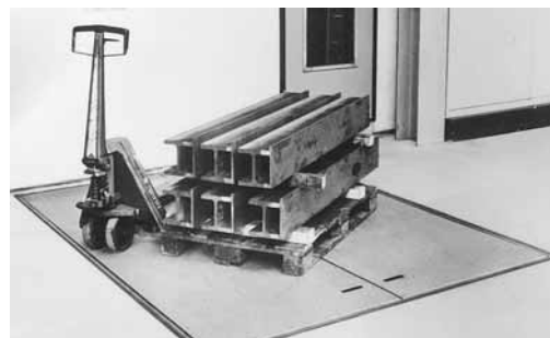
Figura 5: apertura provvista di una botola con portata analoga a quella del pavimento.
