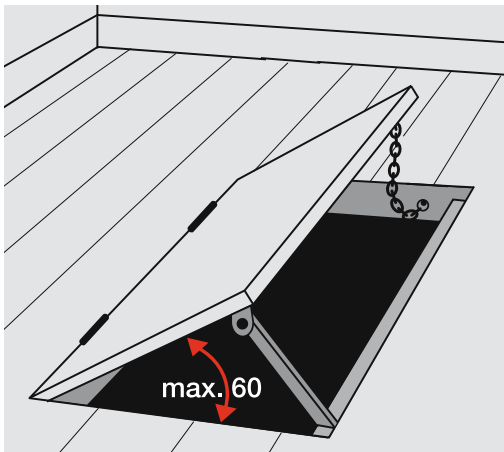
Figura 11: protezione di una botola nel suolo (ad es. per accedere ad un vano raccogli-trucioli) con puntone e catena. La catena è fissata saldamente per impedire che la botola possa cadere all'indietro.
